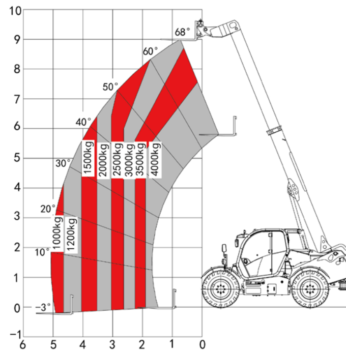
40THCJ09-CU1 Lifting diagram
