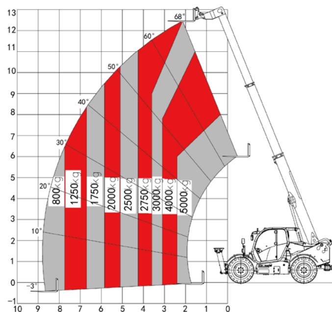
50THCJ13-CU1S Lifting diagram
