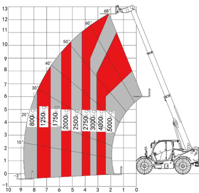
50THCJ13-CU1 Lifting diagram
