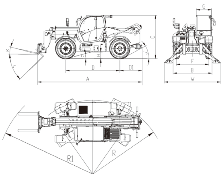
40THCJ09-CU1 Dimension
