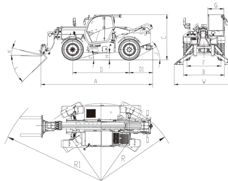
40THCJ13-CU1 Dimension
