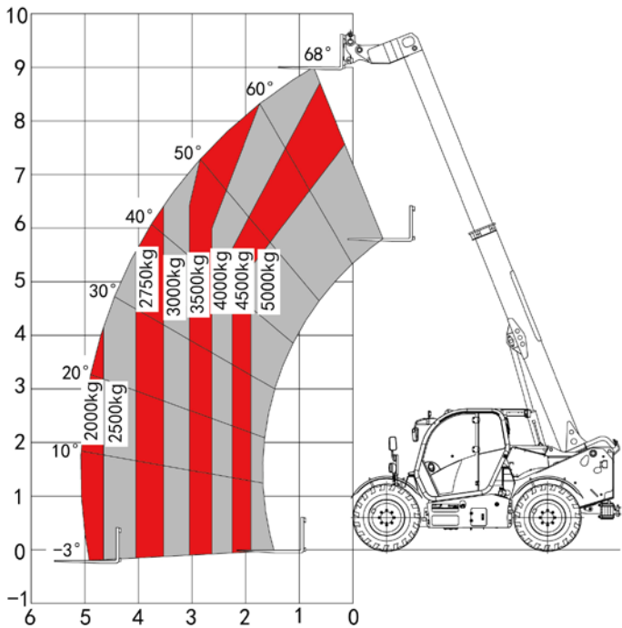
50THCJ09-CU1 Lifting diagram
