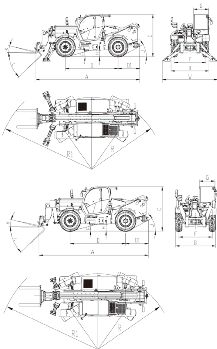
50THCJ13-CU1S Dimension
