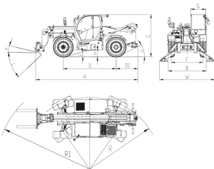
35THCJ09-CU1 Dimension
